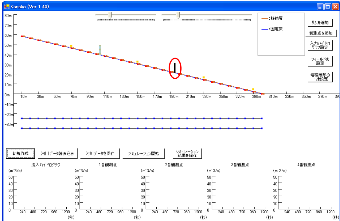
図 8 入力画面（設定を変更する砂防えん堤を選択）
