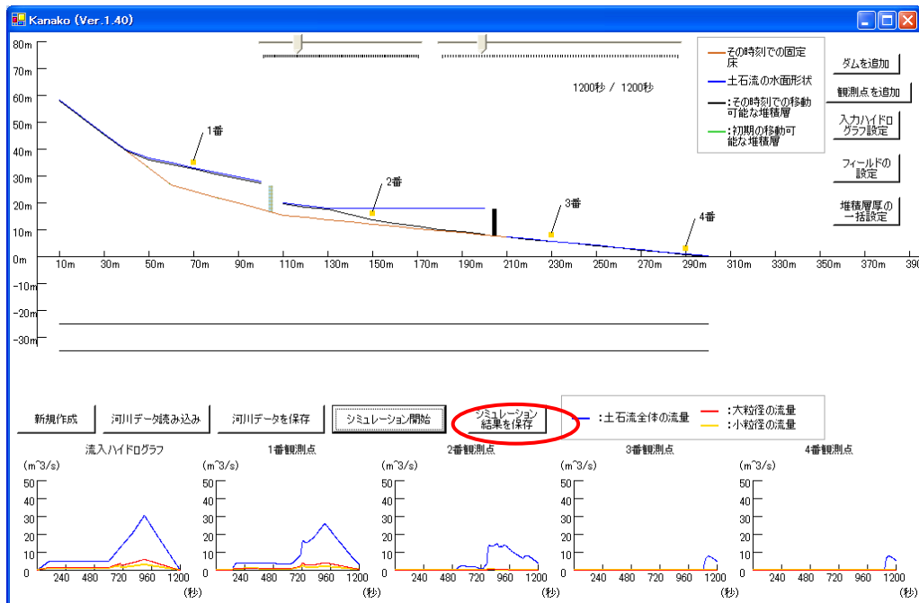
図 70 シミュレーション終了画面
